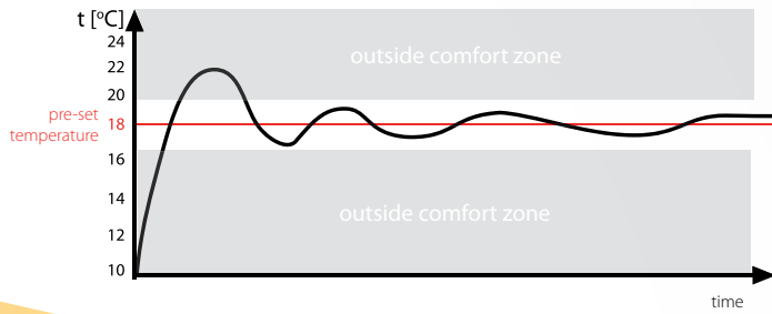
FAN OPERATION DIAGRAM
