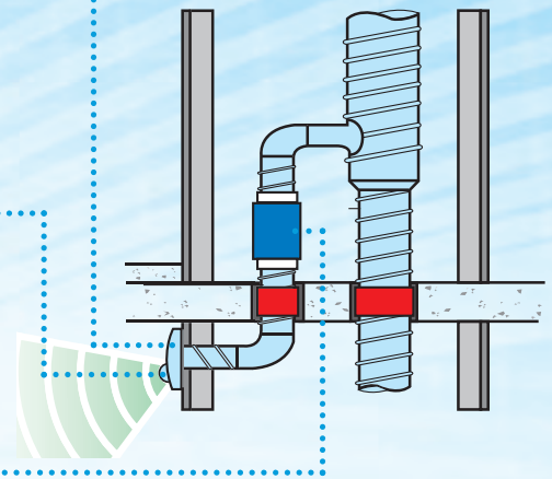
NRG Control Grille/Damper (optional).
