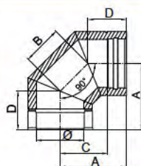
Elbow 90° / DWECO - 60
